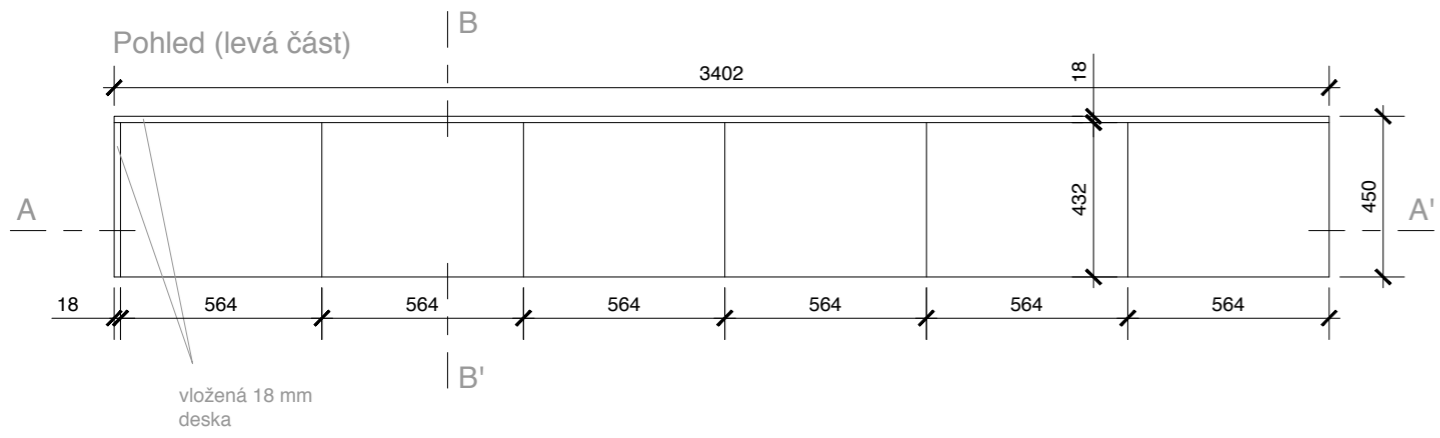
Pohled bez čelních dvířek (levá část)
