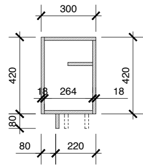
Řez A-A'
